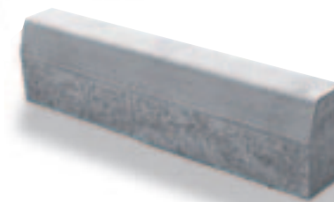
Kiemelt útszegély kopóréteggel Méret: 100 x 25 x 15 cm
