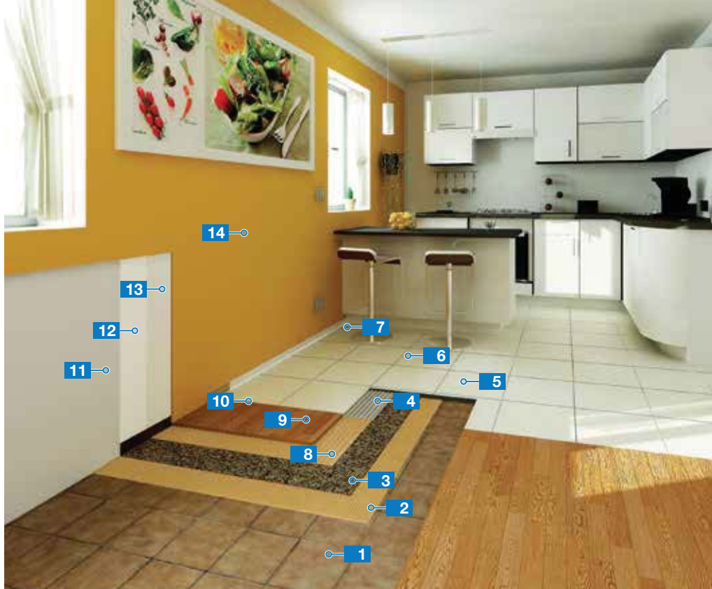
Rendszer meglévő padlóra burkoláshoz hangszigeteléssel
