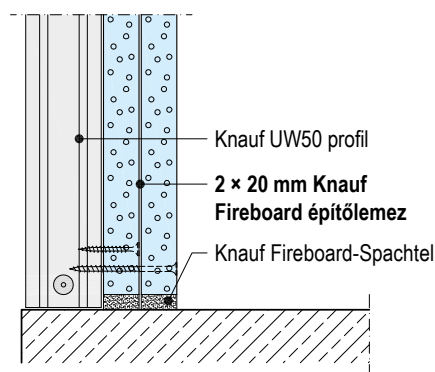
W628-A Aljzatcsatlakozás
