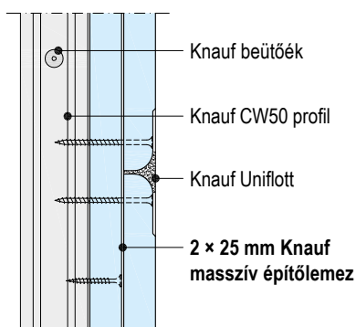
W628-A Lemezillesztés
