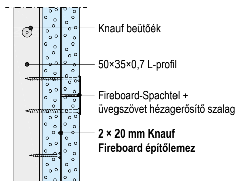
W628-A Lemezillesztés
