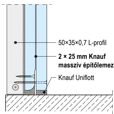
W628-A Aljzatcsatlakozás
