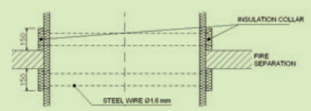
Tűz megállítási kör keresztmetszetű vezeték esetén
