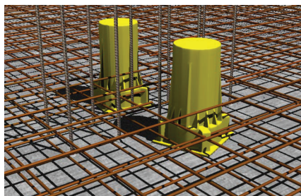
Az FCID szerelése megerősített betonaljzaton
