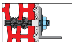
9. lépés - A rögzíteni kívánt elemet csak a kikeményedési idő letelte után csavarja rá a rögzítőszárra.
