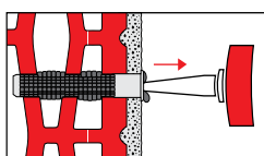
7. lépés - Teljesen töltse ki a furatokat a masszával. A rögzítőszár behelyezésekor a massa a szita-hüvelyen keresztül a tégl üregeibe nyomódik.
