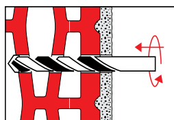
1. lépés - Fúrja ki a megfelelő furatokat.
