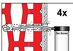
2 és 4 lépés - Portalanítsa a furatokat légpompával.
