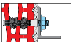
8. lépés - Csavarja bele a masszába a rögzítőszárat a menetnek megfelelő irányban.
