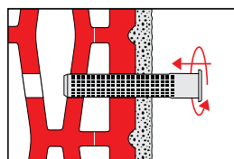
5. lépés - Illesszen szitahüvelyt a furatokba.
