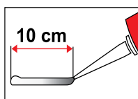
6. lépés - Helyezze a kartust a kinyomópisztolyba, és csavarja rá a keverőszárat. Nyomjon ki kb. 10 cm hosszú csíkot a rögzítőanyagból (ne a furatba), amíg az anyag egyenletesen szürke nem lesz.
