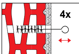
3. lépés - Tisztítsa meg a furatok bel-sejét kefével, hogy a laza por leváljon a felületről.
